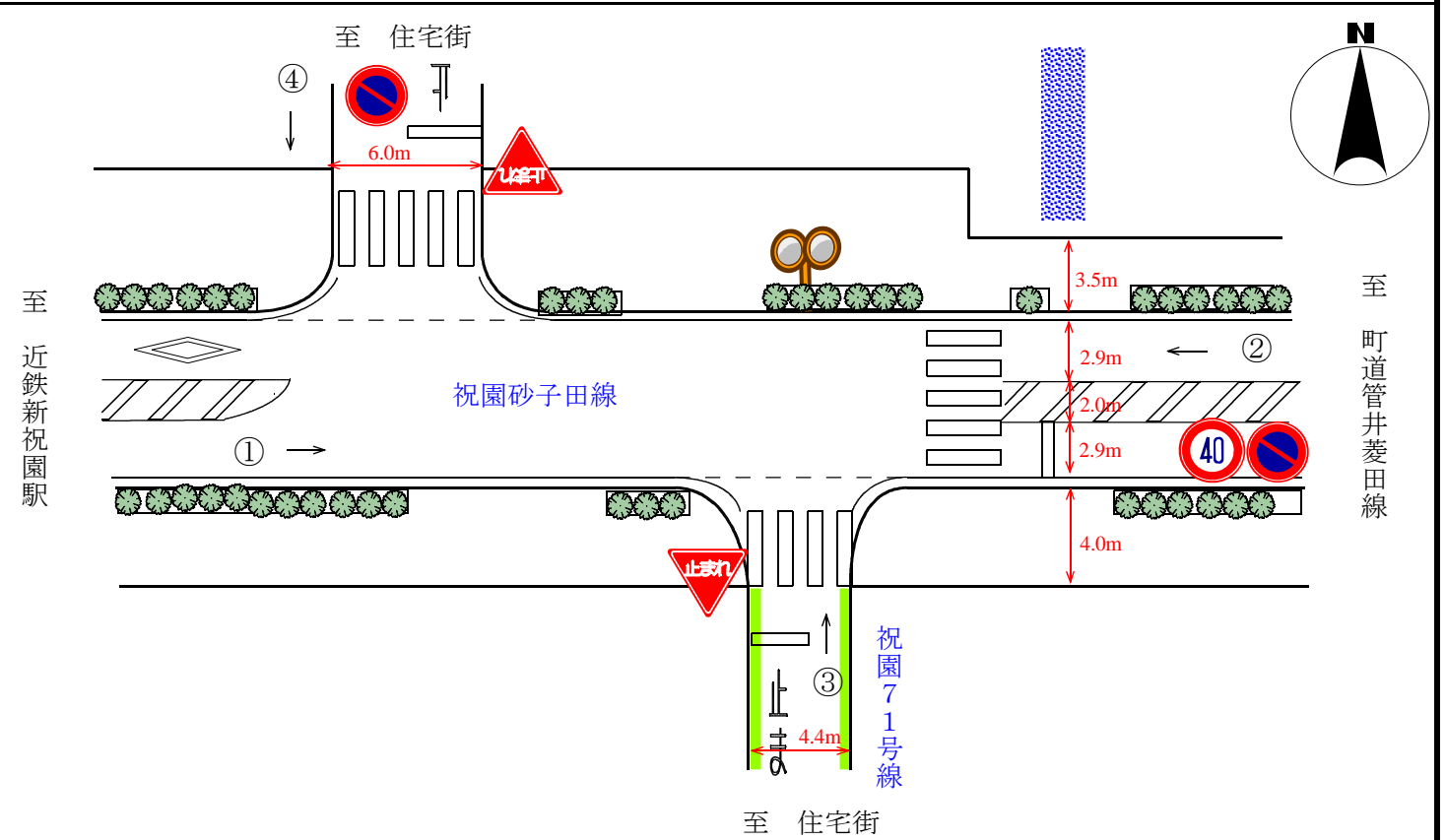
交差点図面
